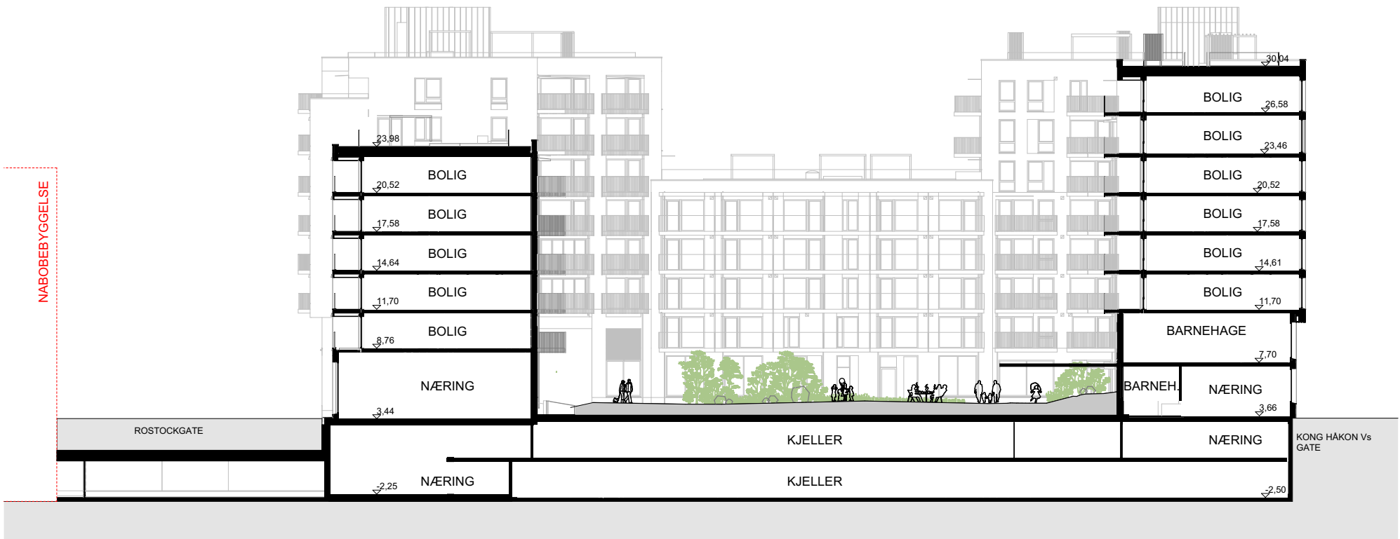
2. Snitt B
