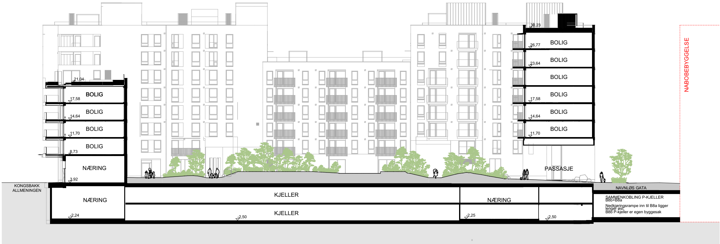
1. Snitt A
