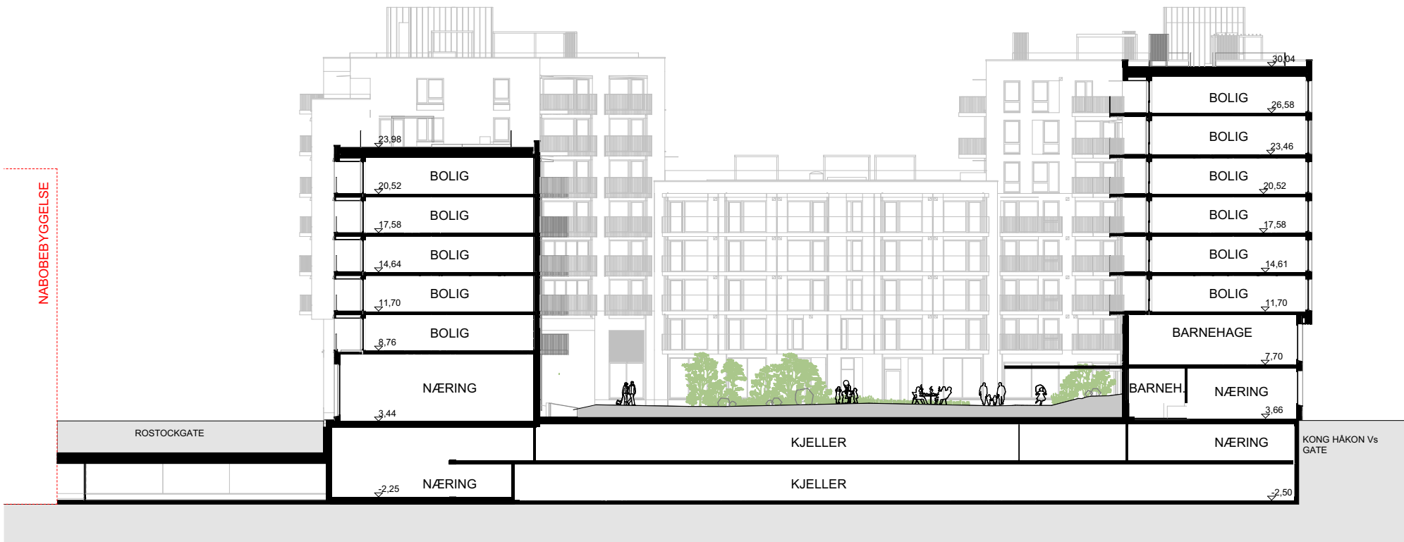
2. Snitt B
