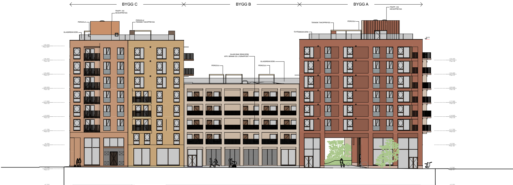
1. Fasade nord
